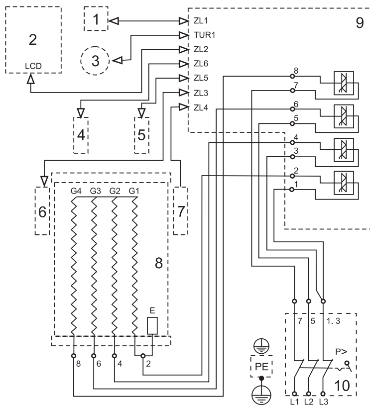
Rys. 7. Schemat ideowy POW-LCD MULTI
